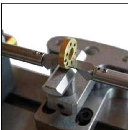
Touches couteaux épaisseur 0.4 mm et table XYZ standard
