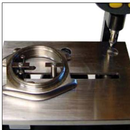
Mesure intérieure en 2 points avec auto-centrage de la pièce sur LVS 50
