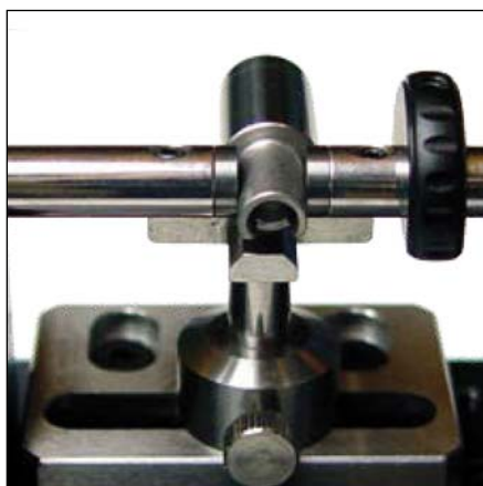
Mesure \varnothing extérieure avec touches \varnothing 6.5 et table XYZ
