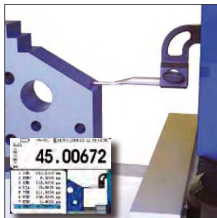
Mesure d'angles et cônes
