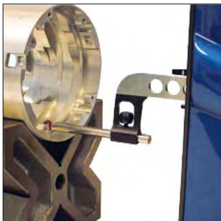
Mesure de diamètres et d'entraxes
