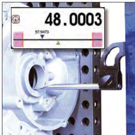
Mesure de diamètres à l'aide d'une touche à bille Ø 2 mm
