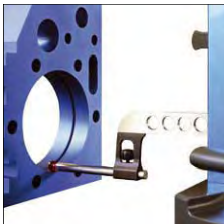
Mesure de diamètres et entraxes
