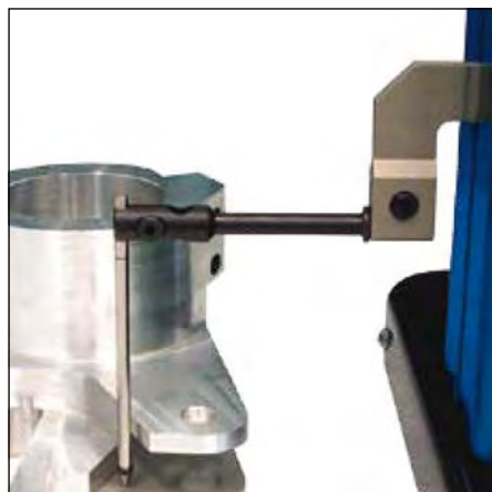
Mesure de profondeurs
