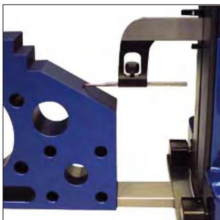
Mesure d'angle
