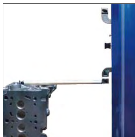
Mesures avec touches jusqu'à 300 mm (sur demande spéciale jusqu'à 500 mm)
