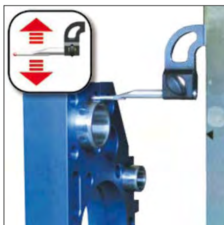
Mesure de diamètres extérieurs automatique avec «TRIMOS® NC movement»
