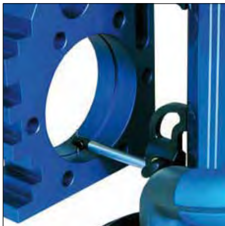
Mesure de diamètres et de profondeur de gorge avec une touche à goupille
