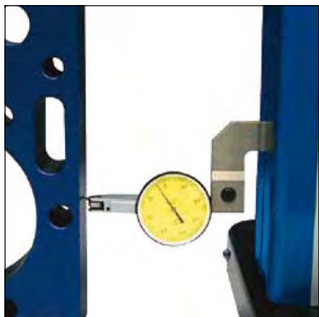
Mesure de perpendicularités
