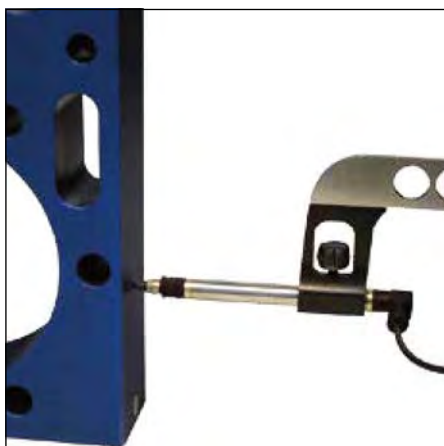
Mesure de perpendicularités avec palpeur électronique
