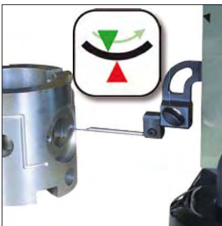
Mesure de petit diamètres avec touche \varnothing 4 mm
