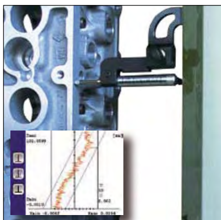
Grâce au palpeur de perpendicularité l'affichage de la courbe et son impression sont possibles
