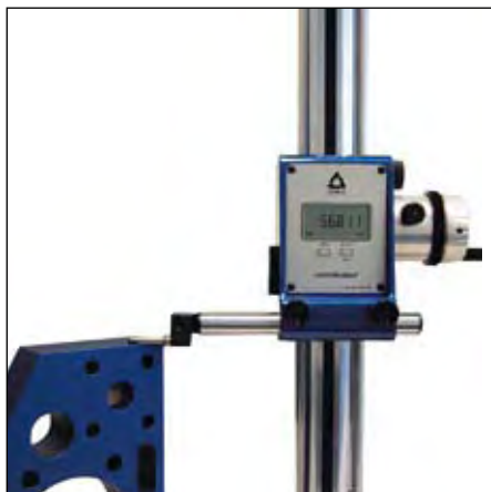
Mesure de hauteurs et de profondeurs
