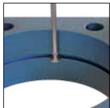
Mesure de rainure intérieure avec accessoires 930.2108, 930.2110 et 905.2205
