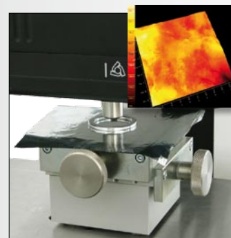
Analyse de la surface d'un film de condensateur
