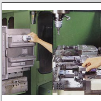
Mesure d'état de surface dans les deux configurations (unité d'avance en place dans l'électronique ou en dehors en utilisant la rallonge)
