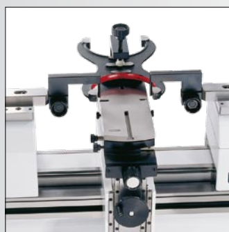
Contrôle de calibres-mâchoires de 12 à 150 mm
