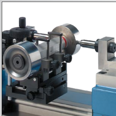
Vérification de tampons lisses
