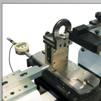
Contrôle de bagues à filetage conique
