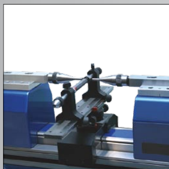
Vérification rapide de tampons lisses avec table flottante
