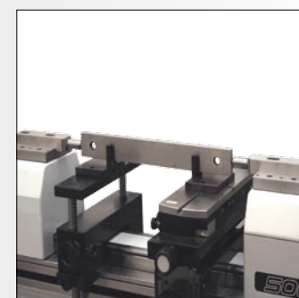
Mesure de cales-étalons
