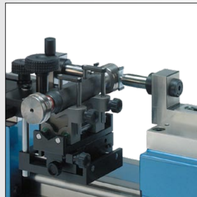
Vérification de tampons filetés
