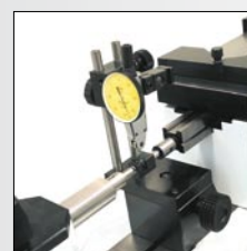
Etalonnage d'indicateurs à levier
