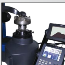
Mesure d'une fraise à plaquettes métal dur
