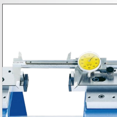
Vérification de pieds à coulisses
