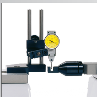
Contrôle de comparateurs à levier
