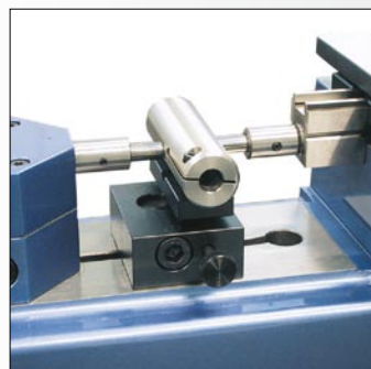
Mesure de diamètres extérieurs
