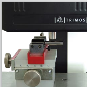
Mesure de rugosité sur un axe rectifié
