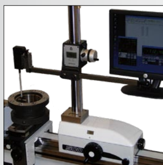
Exécution spéciale pour la mesure de grandes bagues et tampons filetés coniques
