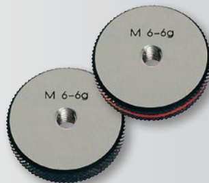
Bagues filetées
