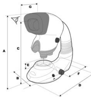
Statif de table de grande stabilité à mise au point intégrée, éclairage diascopique à intensité variable, option de platine flottante.
